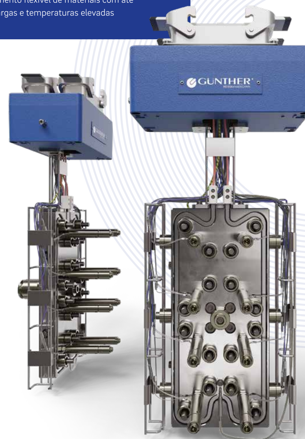
Estrutura do sistema Basic2Connect com bicos do tipo 6 e carburador em "H" de 8 vias
