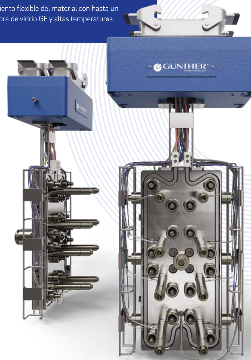
Estructura del sistema Basic2Connect Boquilla tipo 6 Distribuidor en H de 8 elementos
