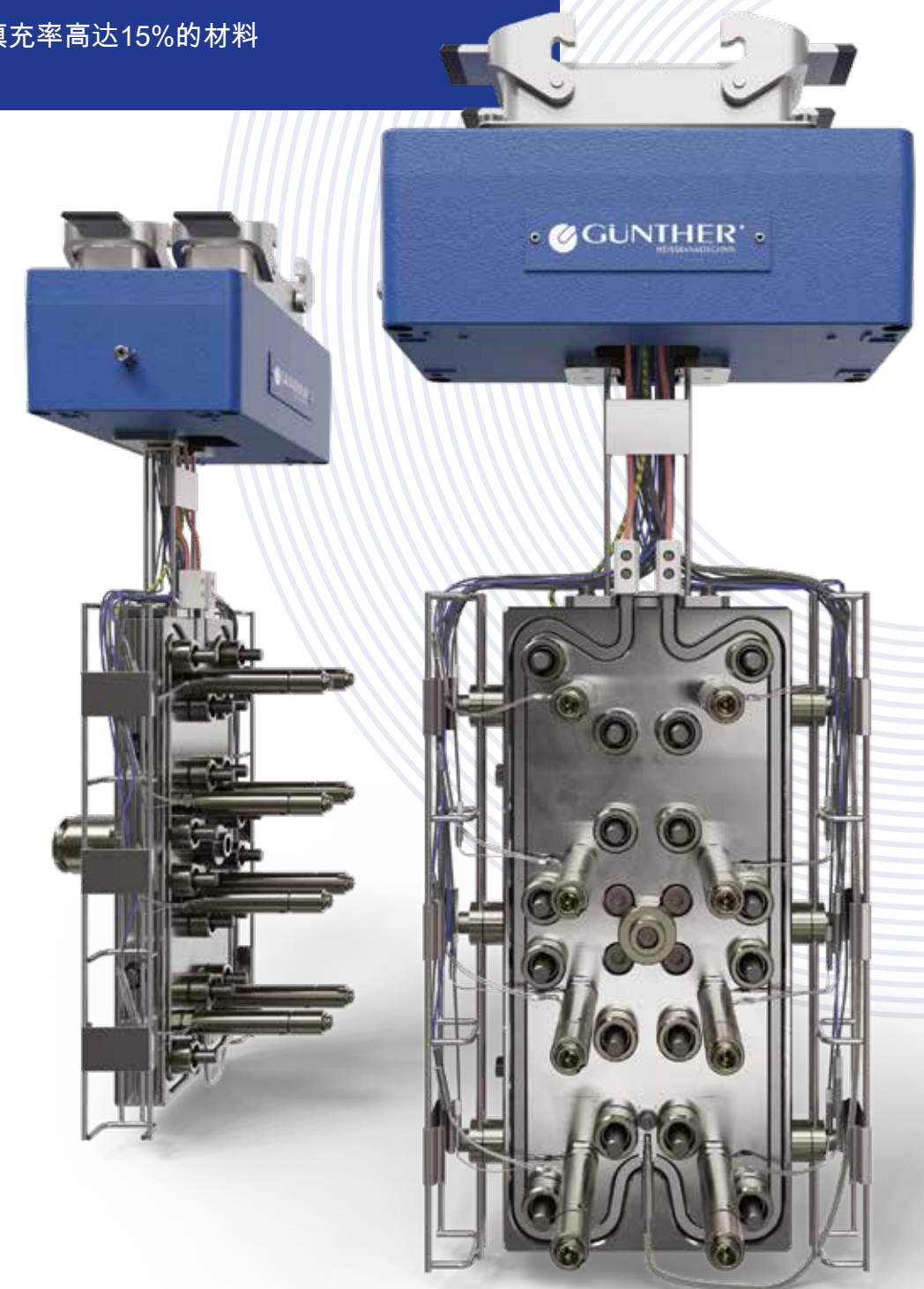
Basic2Connect 系 统6型热嘴 8穴H型分流板
